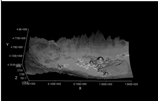
地下水揚水量分布
