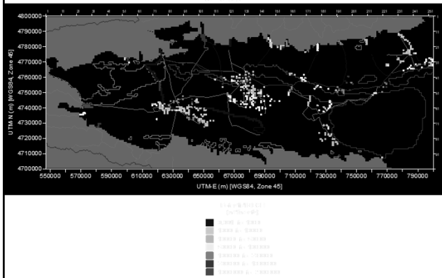
最大地下水涵養量(2003年1月)
