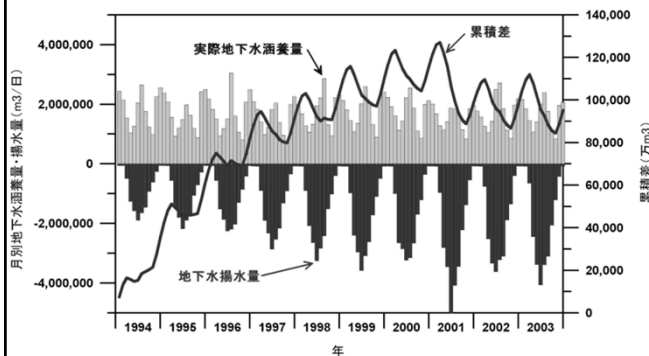
広域三次元モデル地区の 実際地下水涵養量と揚水量および累積差
