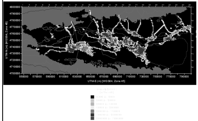
最大地下水涵養量(2003年7月)
