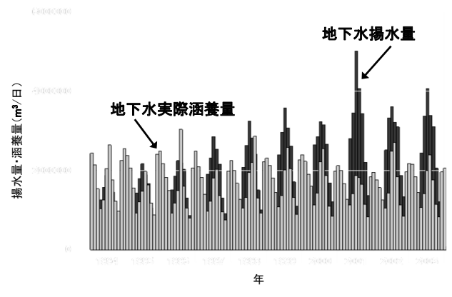
月別地下水揚水量と涵養量
