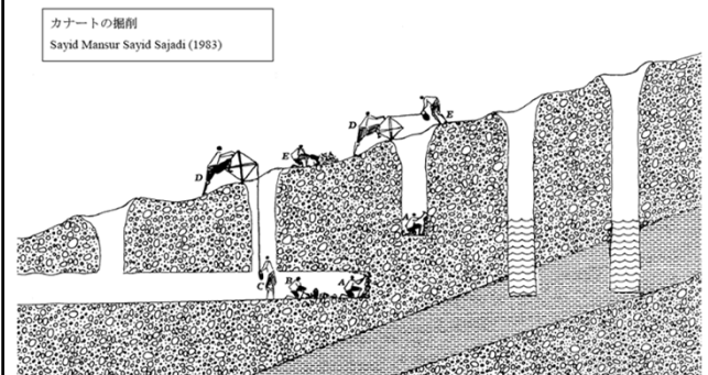
カナートの掘削方法
