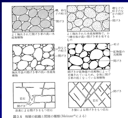
図 3.6 地層の組織と間隙の種類 (Meinzer による)
