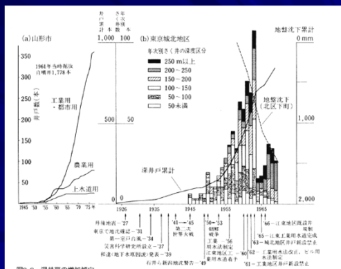
図2-9 深井戸の増加傾向 (a) 東北農政局・山形市 b. 水収支研究グループ「地下水量の管理」東海大学出版会, 1976による)
