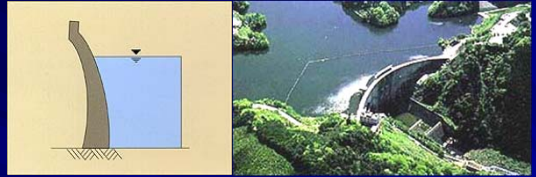
青蓮寺ダム(水資源開発公団)
