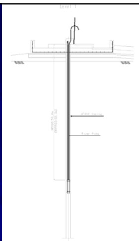
足踏み式人力 ポンプ井戸の 構造
